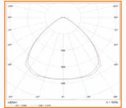
98 Derece / 98 Degrees
