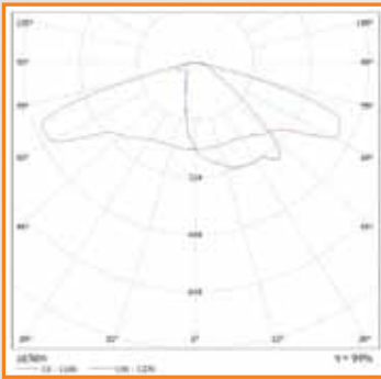
Asimetrik / Asymmetric
